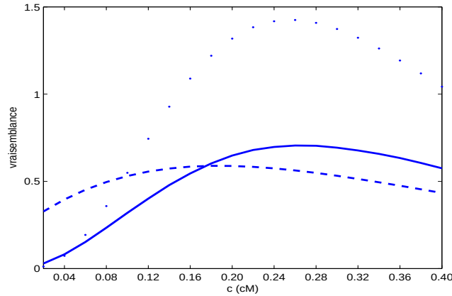
FIG. 6.1 – Courbes de vraisemblance \mathcal{L}^{(MC)}(c, t, N, \pi^0 | n) (ligne continue), \mathcal{L}^{(1)}(c, t, N, \pi^0 | n) (points), et \mathcal{L}^{(KBE)}(\rho, \tau, \pi^0 | n) (ligne en pointillés) en fonction de c . On a N = 10000 , t = 100 , \pi^0 = (0.21, 0, 0.37) et n = (29, 3, 58, 59) . Pour \mathcal{L}^{(MC)}(c, t, N, \pi^0 | n) on simule M = 300 populations pour chaque valeur de c .
