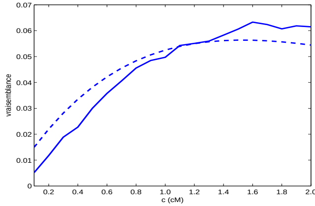
FIG. 6.2 – Courbes de vraisemblance \mathcal{L}^{(MC)}(c, t, N, \pi^0 \mid n) (ligne continue) et \mathcal{L}^{(KBE)}(\rho, \tau, \pi^0 \mid n) (ligne en pointillés) en fonction de c . On a N = 250 , t = 50 , \pi^0 = (0.21, 0, 0.37) et n = (30, 5, 65, 50) . Pour \mathcal{L}^{(MC)}(c, t, N, \pi^0 \mid n) on simule M = 2000 populations pour chaque valeur de c .
